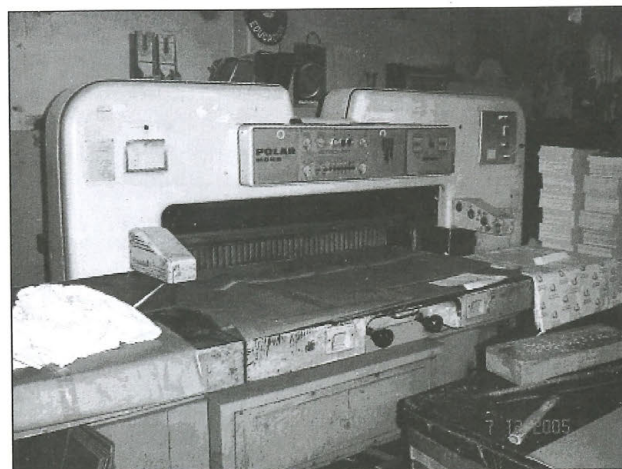
Guillotinas: En algunos talleres se encuentran operando sin sensores que impidan su accionamiento cuando el operador aún tiene las extremidades en la zona de corte.
