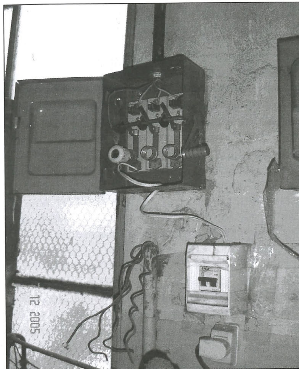
Se han detectado tableros eléctricos sin cerrar, al alcance del personal, con los bornes y llaves energizadas expuestas, cableado que no está adecuadamente contenido y nuevas conexiones improvisadas. Gran parte de la instalaciones carecen de "puesta a tierra" y los disyuntores diferenciales son prácticamente inexistentes.
